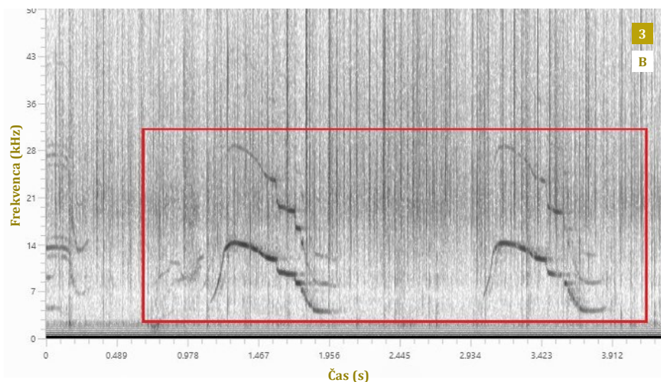
Spektrograma oglašanja delfinov pred Piranom. Znotraj rdečih okvirjev sta primera dveh različnih podpisnih žvižgov (A, B), posnetih s pomočjo hidroфона.
